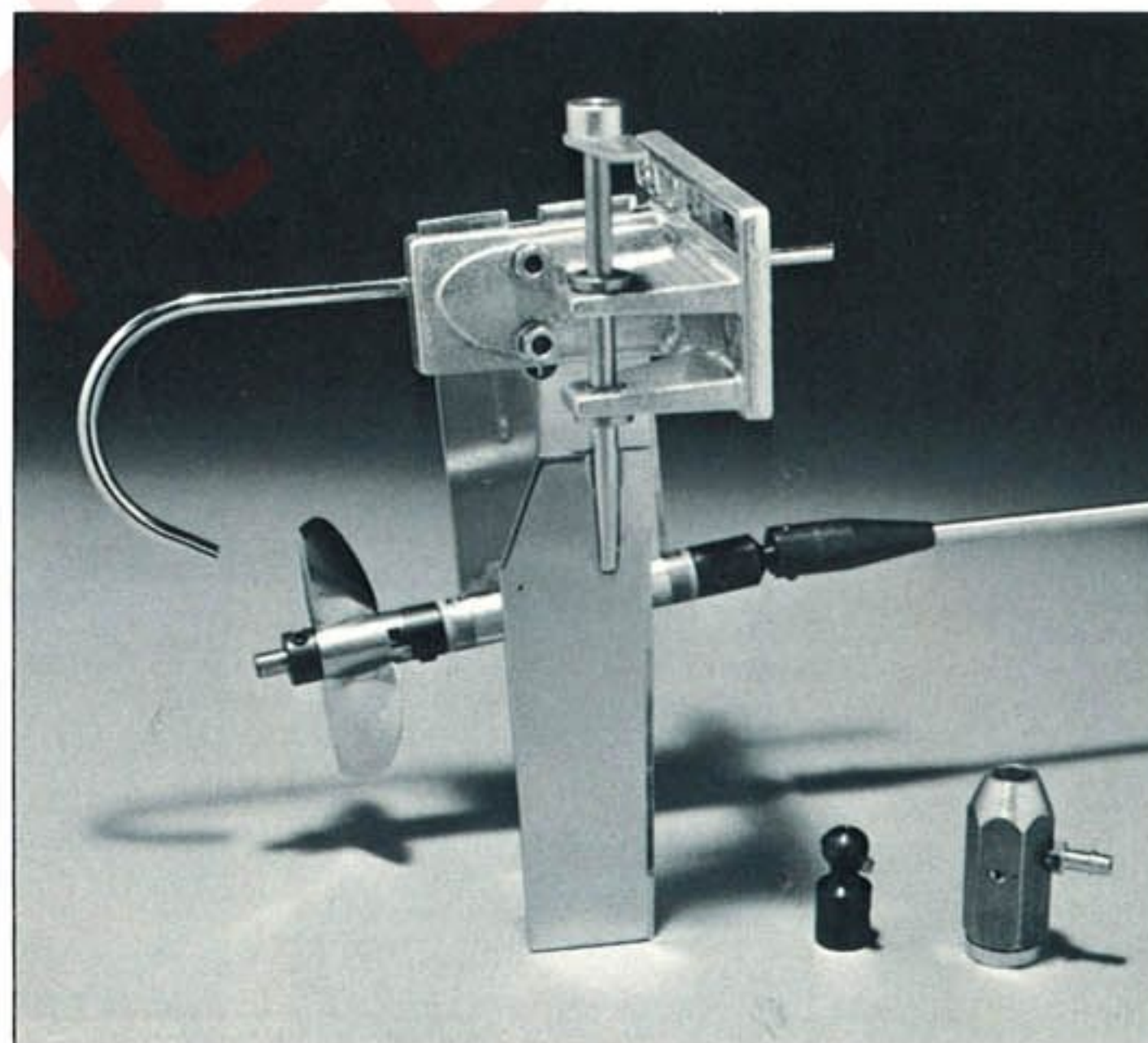
写真(右)スーパー・エンジンパーツセット 40用 ダイヤモンド研磨仕上げの光沢あるフライホイール、精密なジョイント軽く丈夫なエンジン・マウントのセット(各エンジン用あり) 写真(左)スーパー・スクリューセット(ハイドロ)40用 アウト・ドライブ・アセンブリーで船外からブラケットの上・下の位置及びスラスト角と、左・右の角度を変更できます(PAT. PENDING)シャフトは焼入れ研磨加工済のセットです。 写真(上)スーパー・スクリューセット(モノ)40用 ボールジョイント、軸受けメタル、スタンチューブ、シャフト、ステンレスブラケット、ラダー
