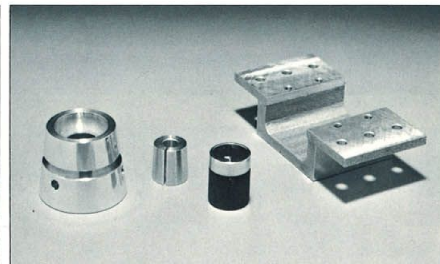
写真(右)スーパー・エンジンパーツセット 40用 ダイヤモンド研磨仕上げの光沢あるフライホイール、精密なジョイント軽く丈夫なエンジン・マウントのセット(各エンジン用あり) 写真(左)スーパー・スクリューセット(ハイドロ)40用 アウト・ドライブ・アセンブリーで船外からブラケットの上・下の位置及びスラスト角と、左・右の角度を変更できます(PAT. PENDING)シャフトは焼入れ研磨加工済のセットです。 写真(上)スーパー・スクリューセット(モノ)40用 ボールジョイント、軸受けメタル、スタンチューブ、シャフト、ステンレスブラケット、ラダー
