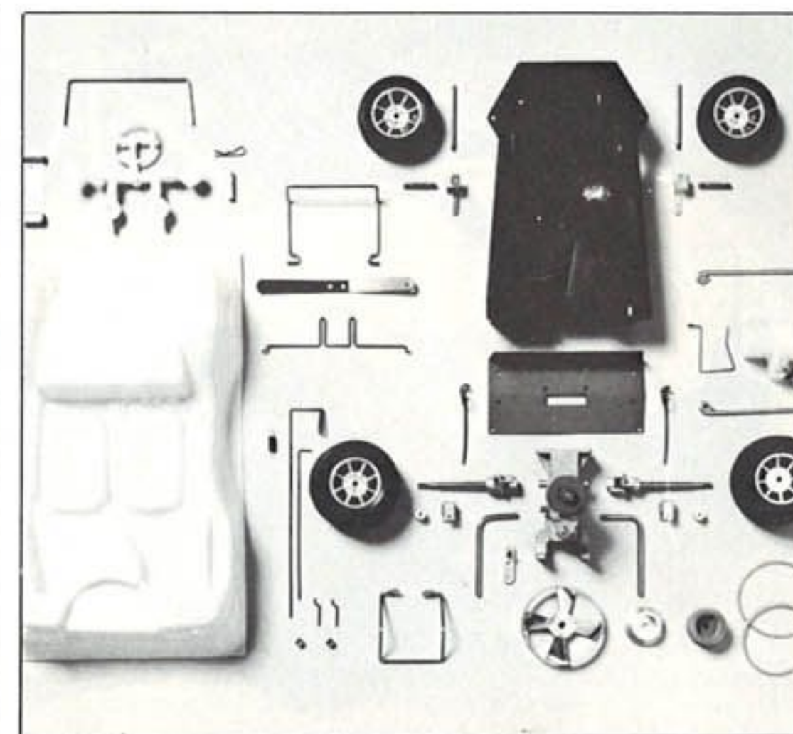
ピーナッツ09バギー部品一式
