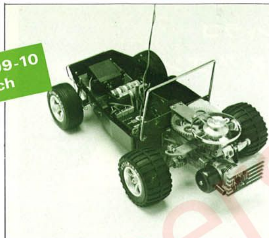
スタビライザー付リアサスペンション
