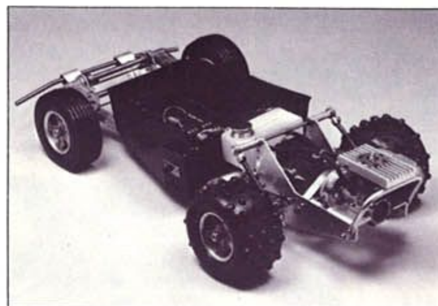
防水と、防塵の取り付けやすいメカボックス。各社のメカが取り付けられる。特製燃料タンクで、一段と性能アップ。
