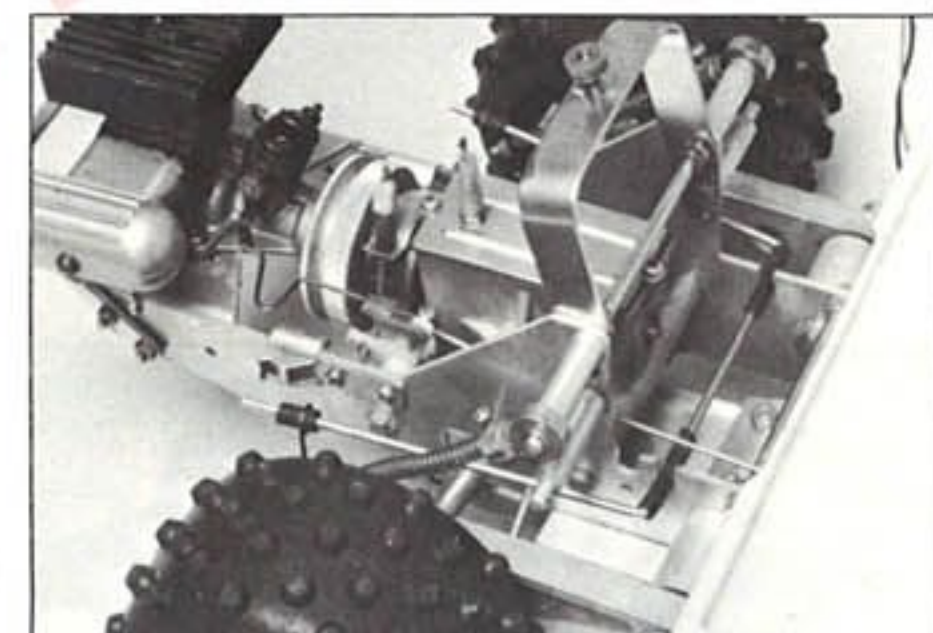
すべて工場完成部品の精密ダイカスト部品、オイルバス式密閉式ギヤボックス。グリップカのあるものすごいポタイヤ。
